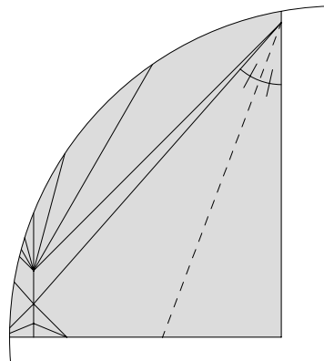
20. Marquer la bissectrice.
